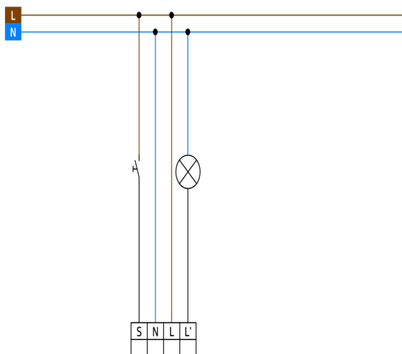
Wiring diagramms
