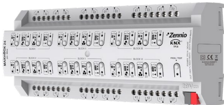
ZIO-MB24 (90 x 60 x 210 мм)
