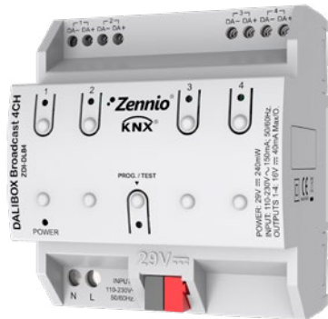
ZDI-DLB4 (90 x 60 x 80 мм)
