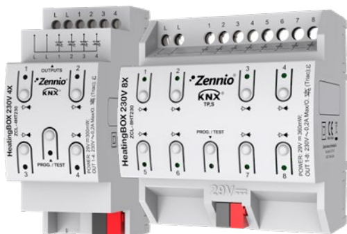
ZCL-4HT230 (90 x 67 x 35 мм)
