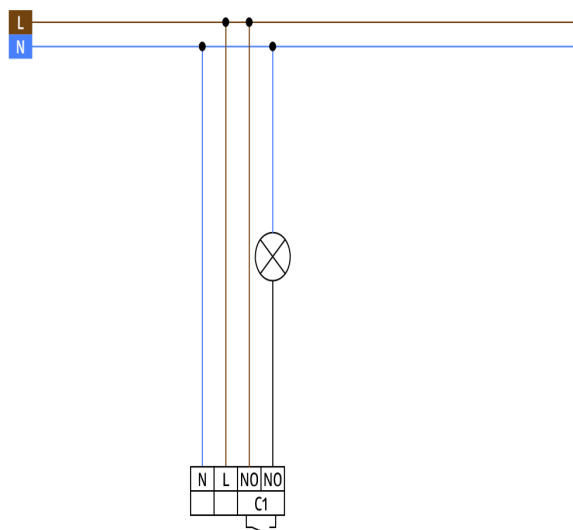
Wiring diagramms
