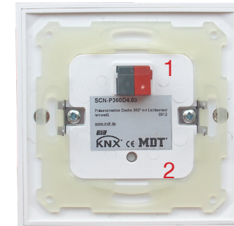
SCN-P360x3.03 Rückansicht - Back view
